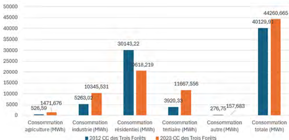
Figure 25 : Comparaison de la consommation d'énergie par secteur entre 2012 et 2023 (Source : PCAER)
