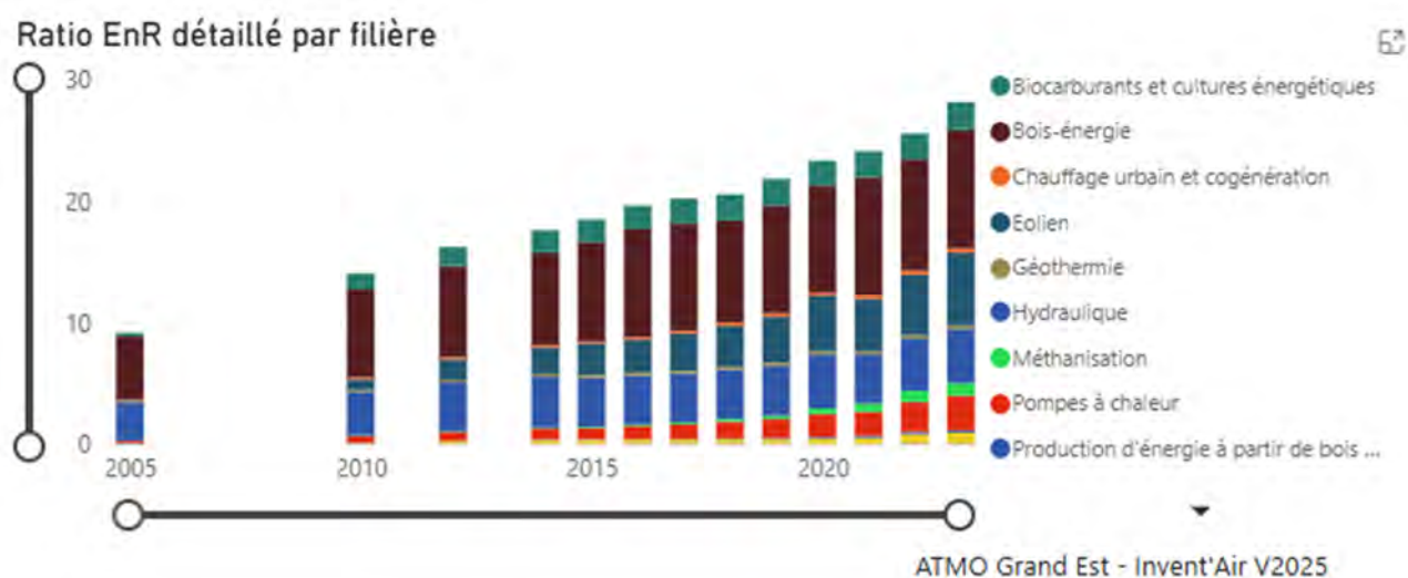
Figure 36 : Ratio d'ENR par filière entre 2005 et 2023 sur la CC3F (Source : ATMO Grand Est)
