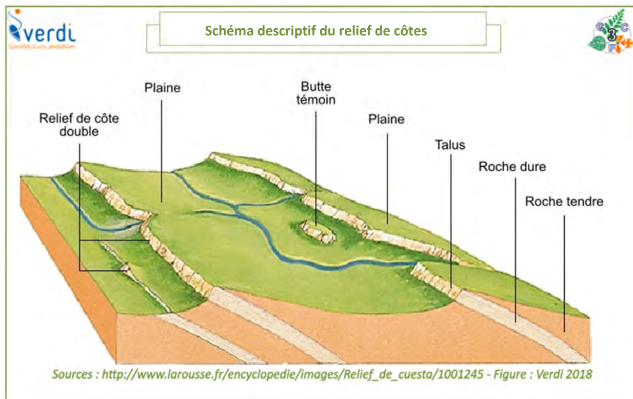
Figure 3 : Schéma descriptif du relief de côtes
