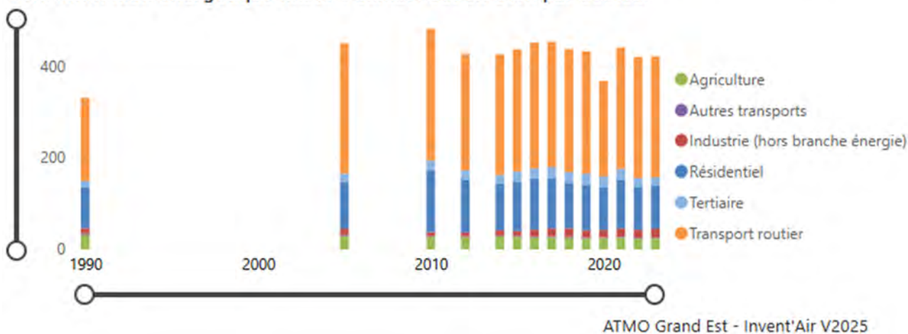
Figure 28 : Consommation énergétique final a climat réel de la CC3F par secteur entre 1990 et 2023
